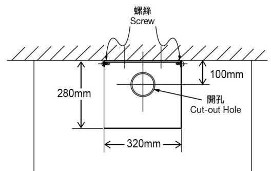
俯視圖 Top View
