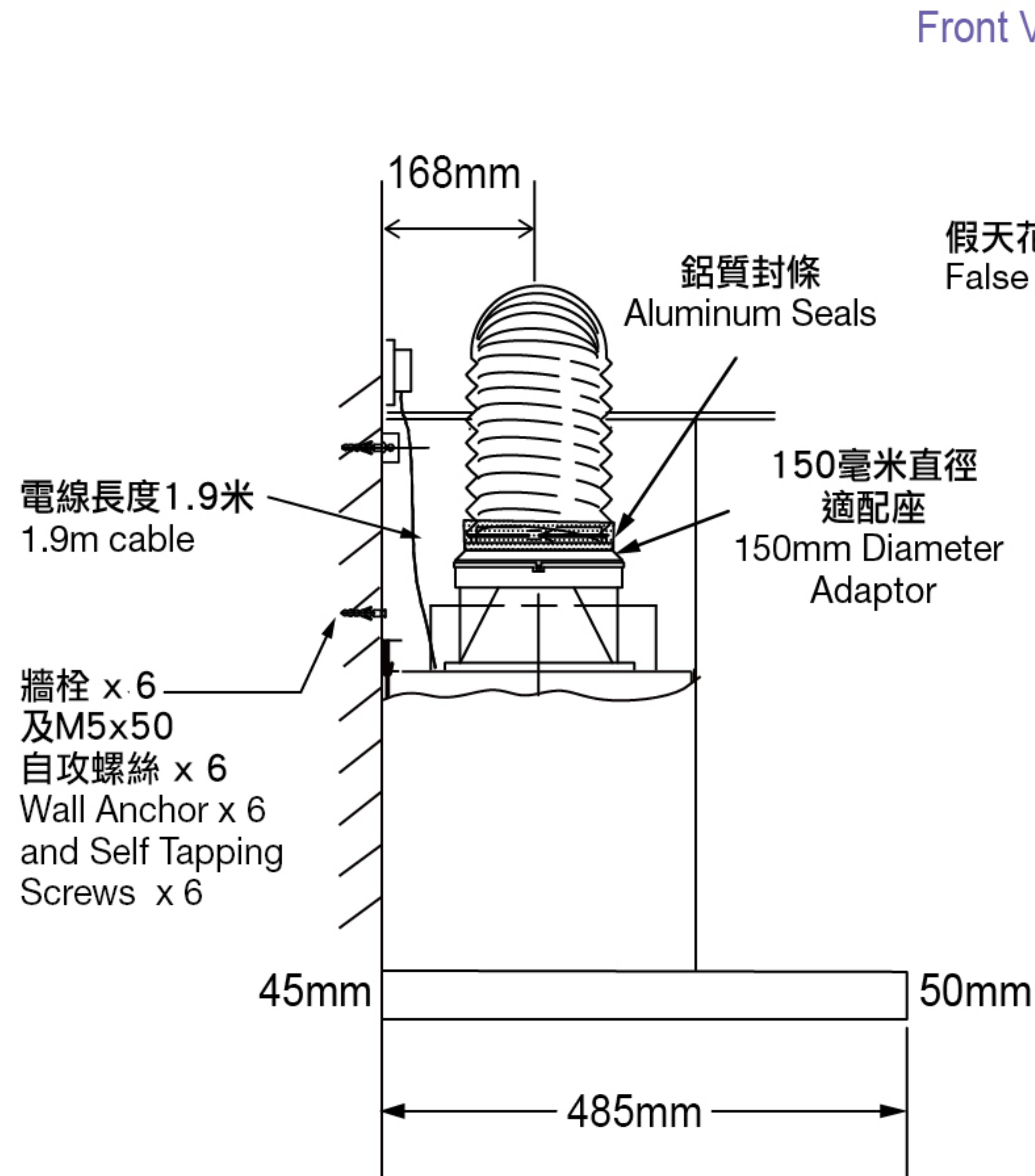
正視圖 Front View
