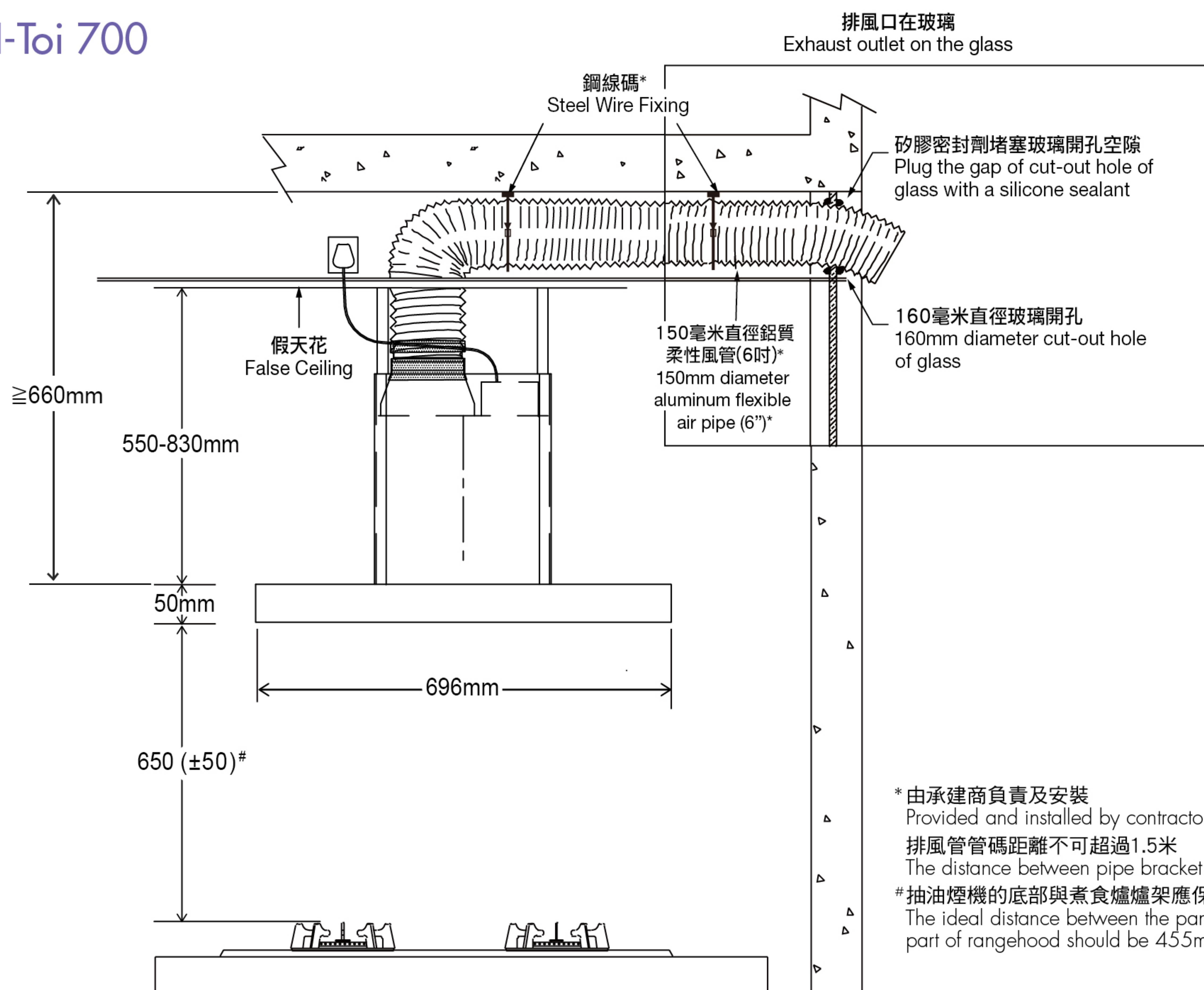
正視圖 Front View
