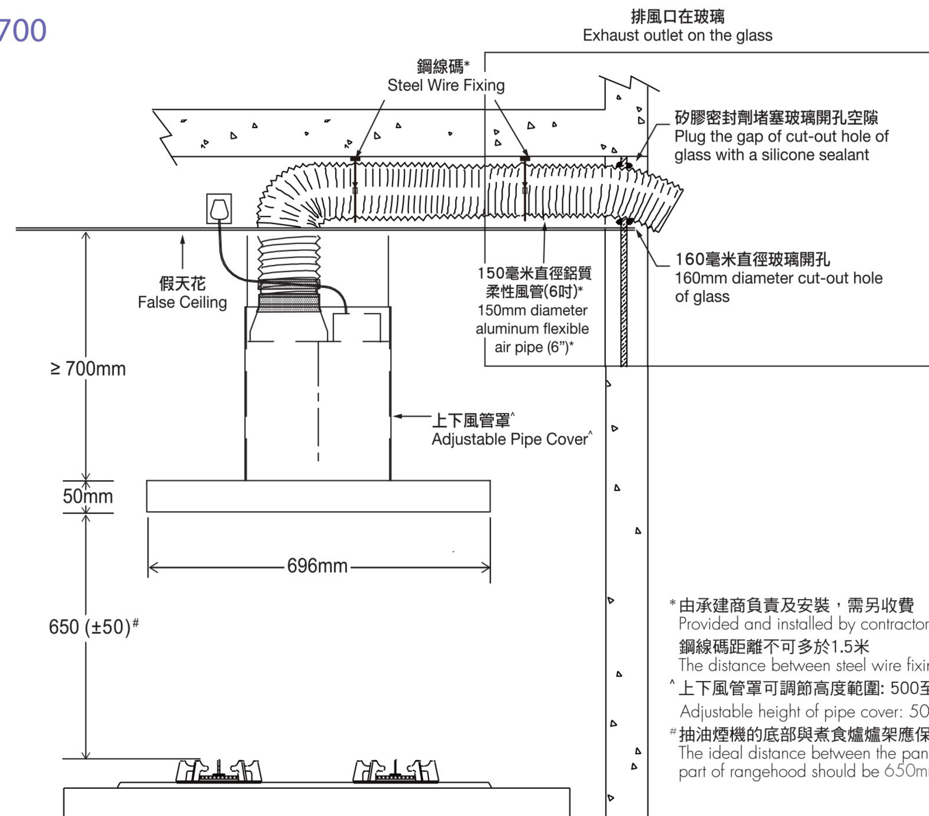
正視圖 Front View
