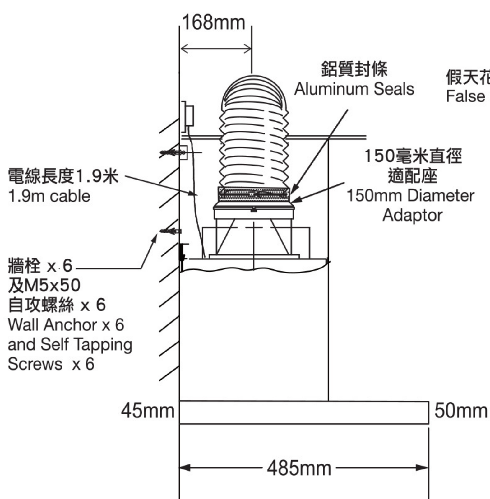
側視圖 Side View
