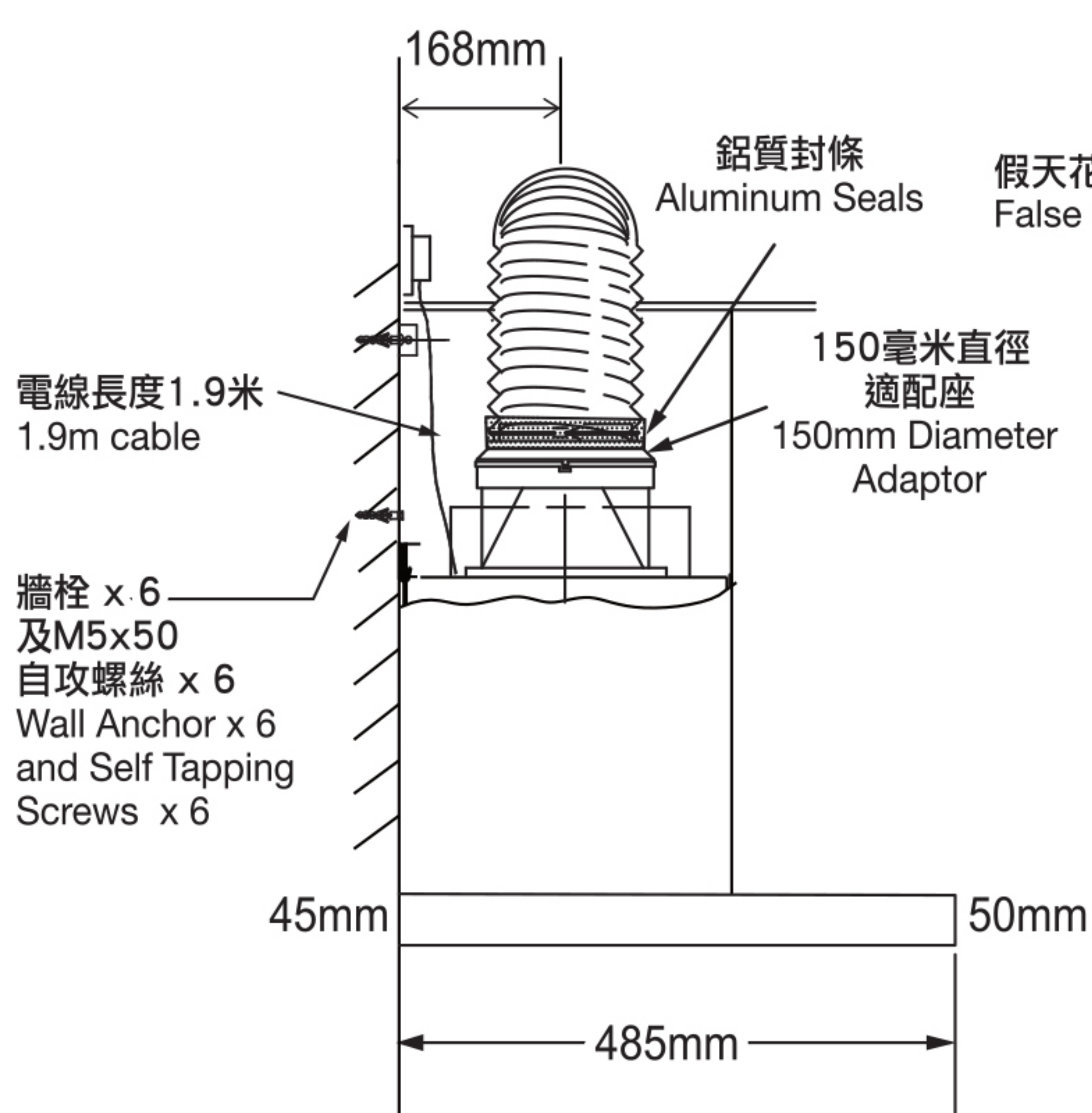
側視圖 Side View
