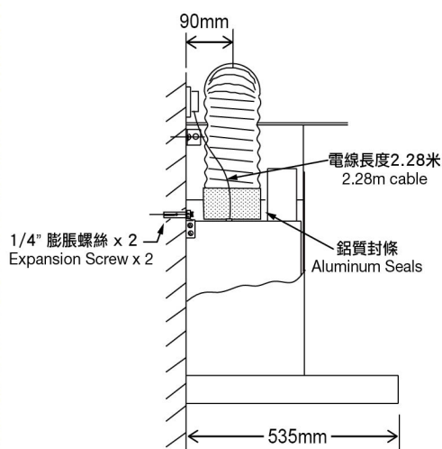
側視圖 Side View
