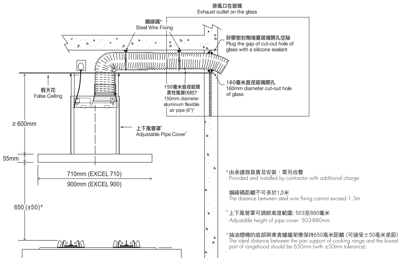
正視圖 Front View
