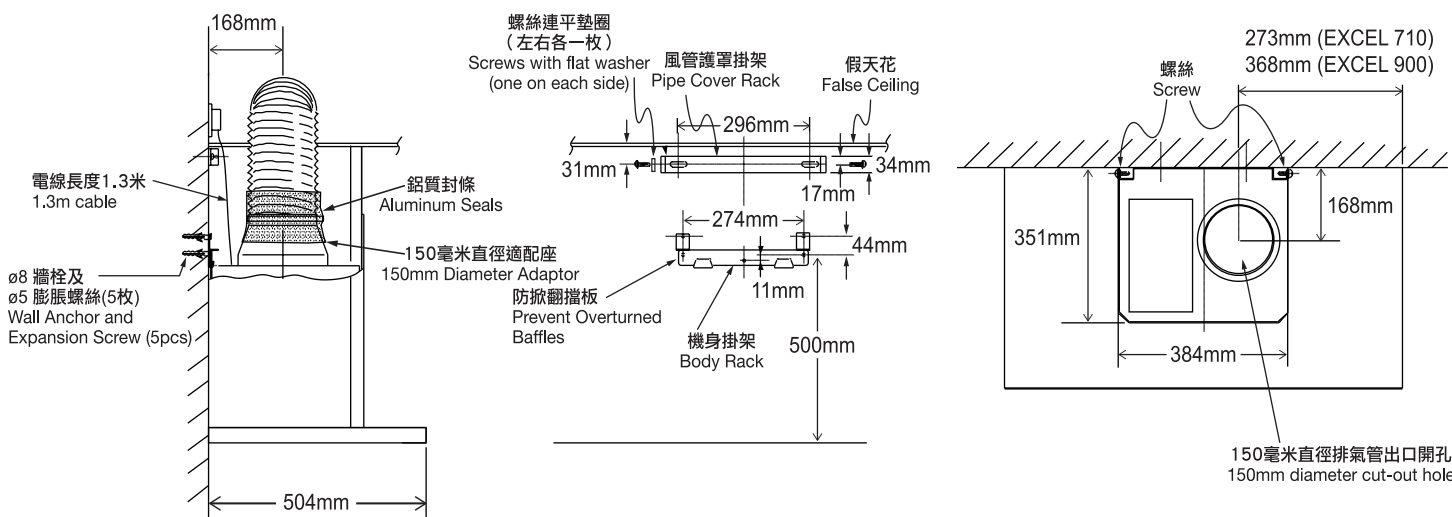
側視圖 Side View
