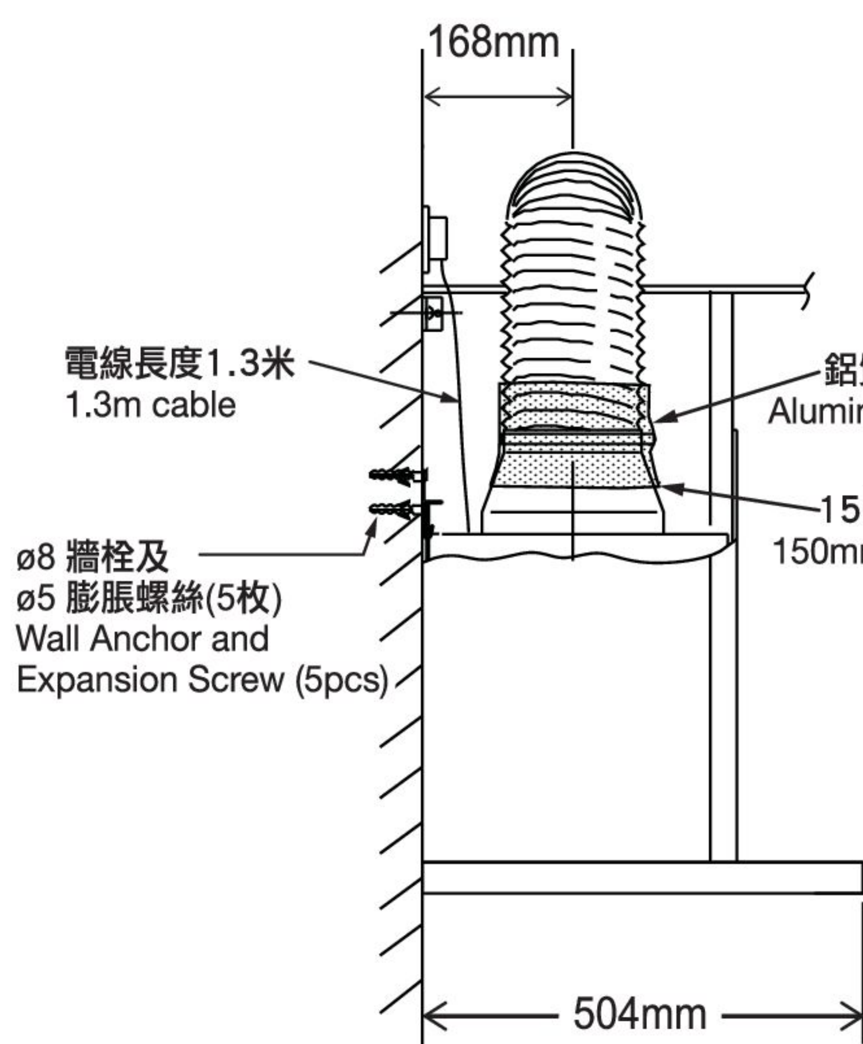
側視圖 Side View
