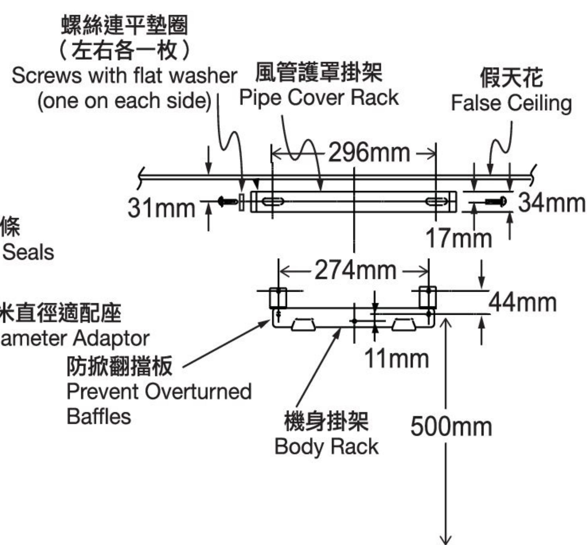
正視圖 Front View
