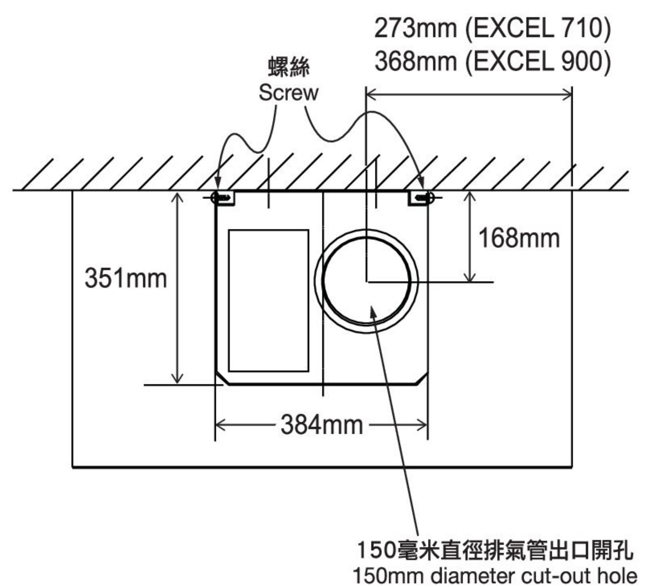
俯視圖 Top View
