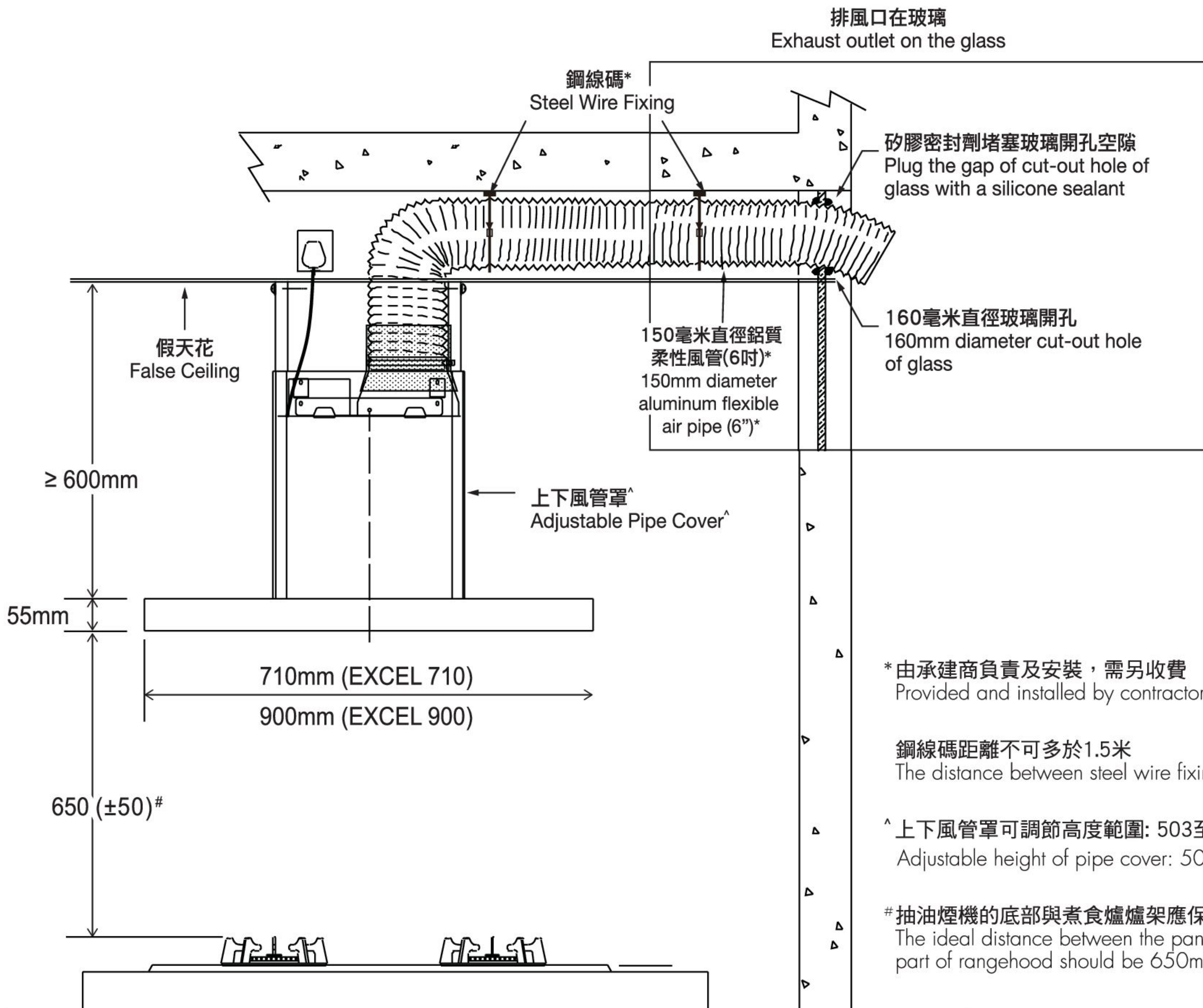
正視圖 Front View
