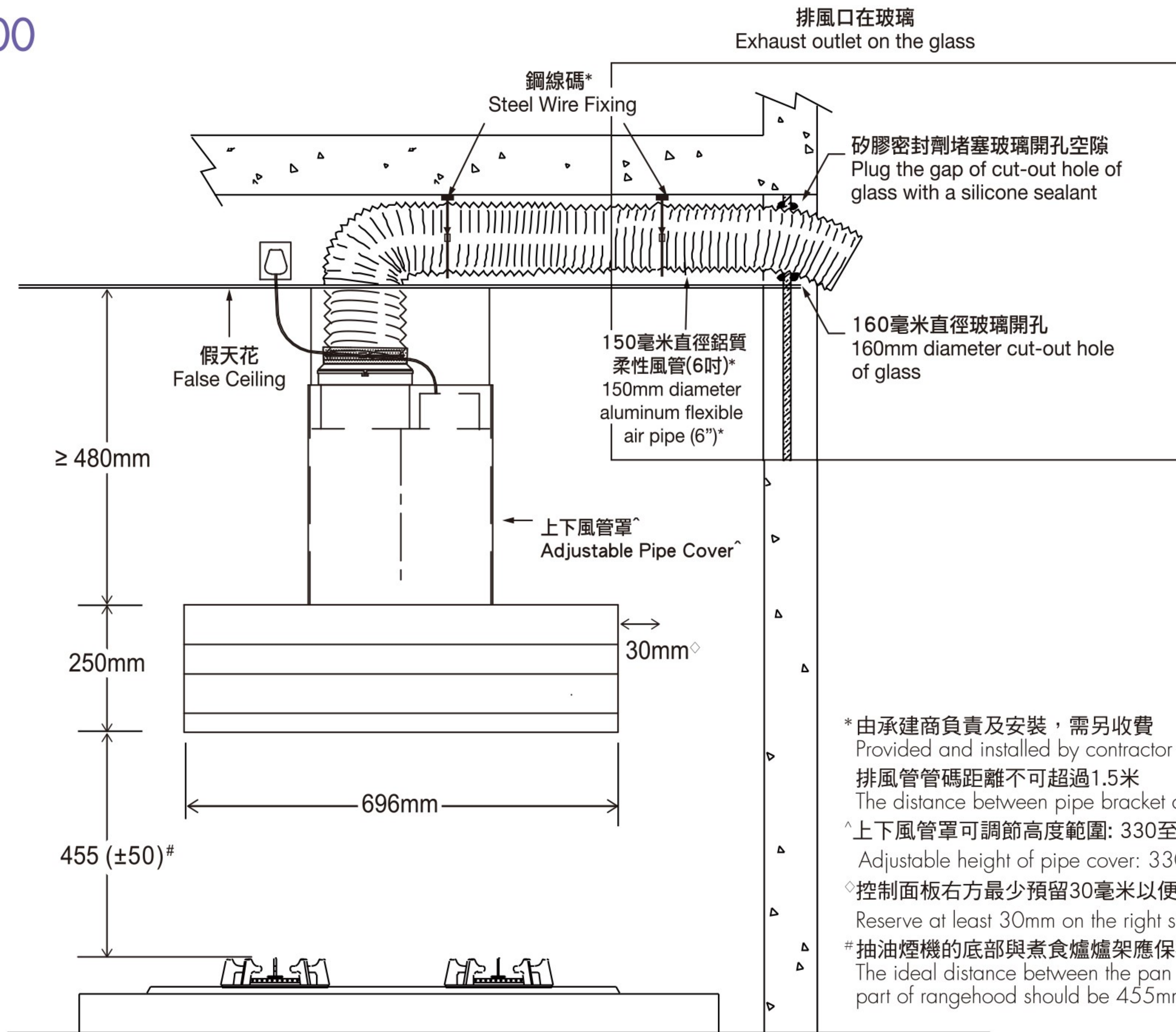
正視圖 Front View
