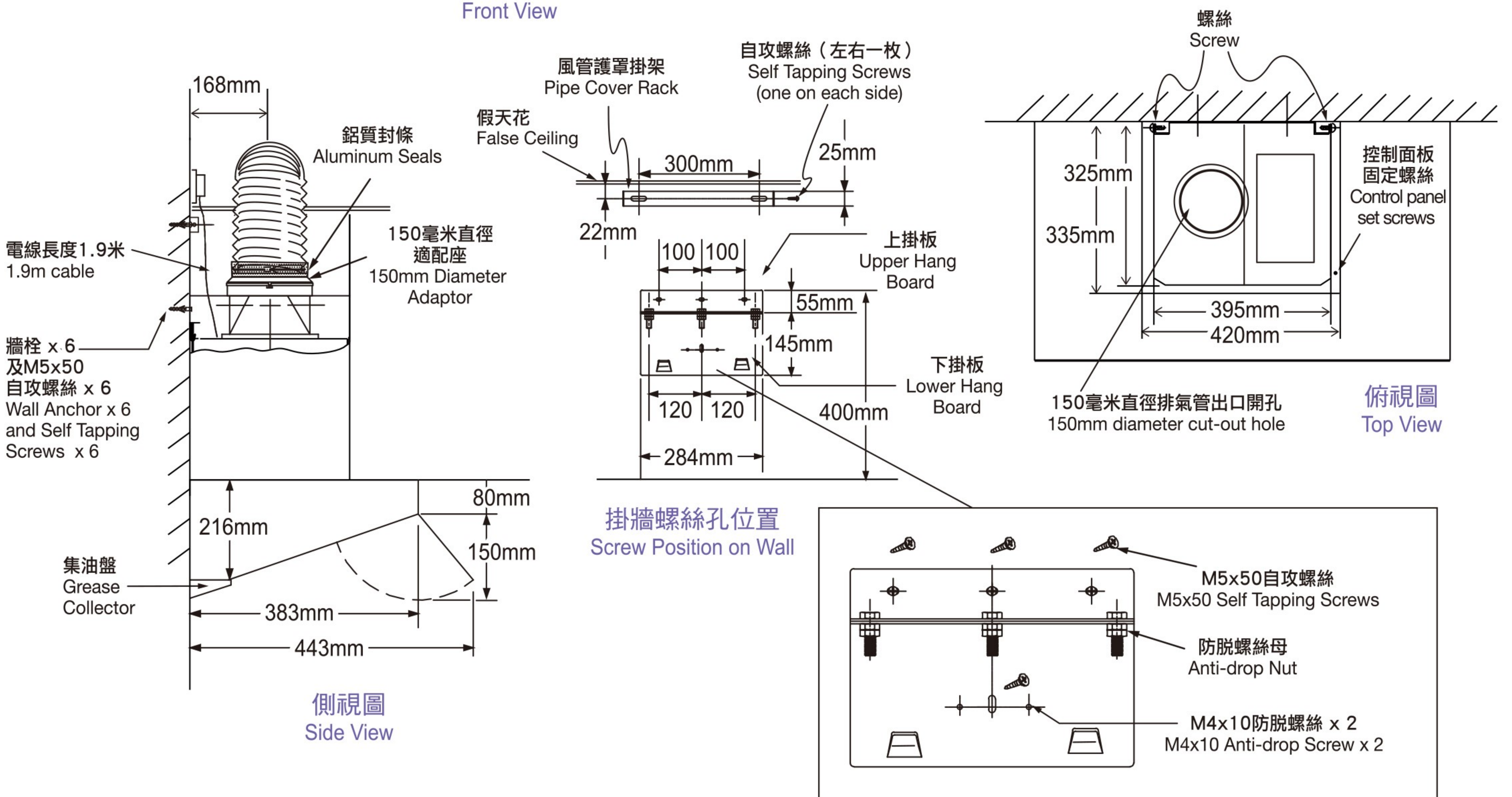
正視圖 Front View
