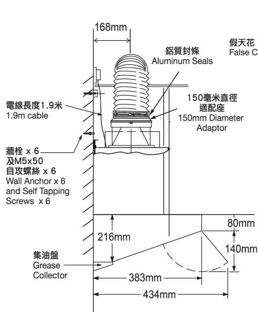
側視圖 Side View
