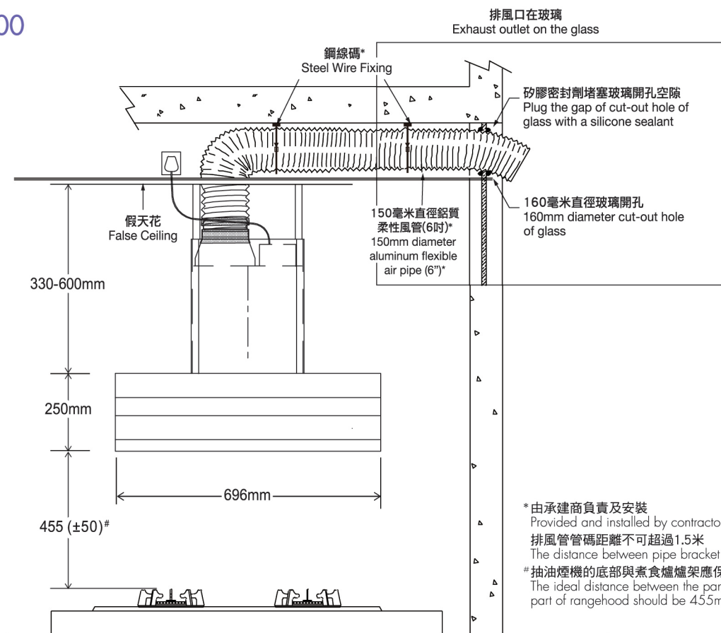
正視圖 Front View
