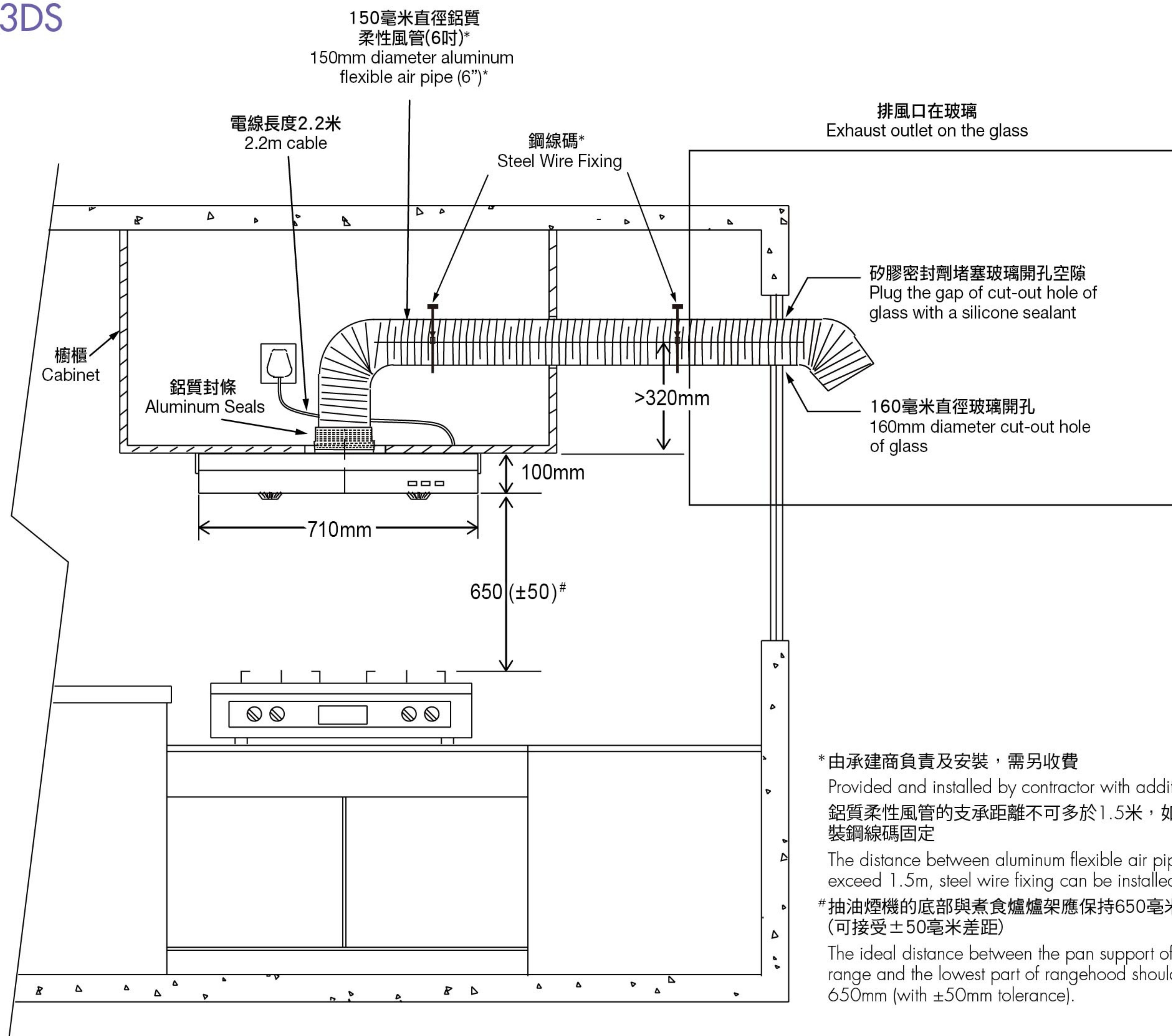
正視圖 Front View
