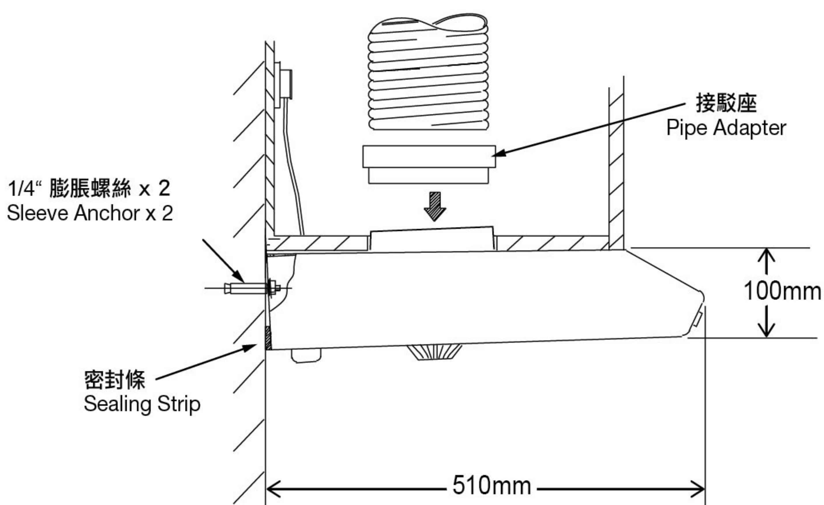
側視圖 Side View
