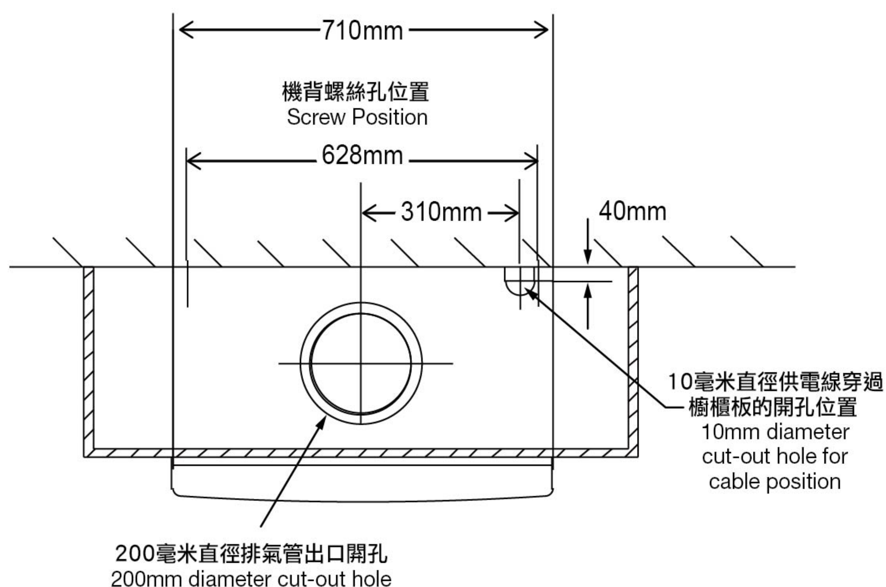
俯視圖 Top View
