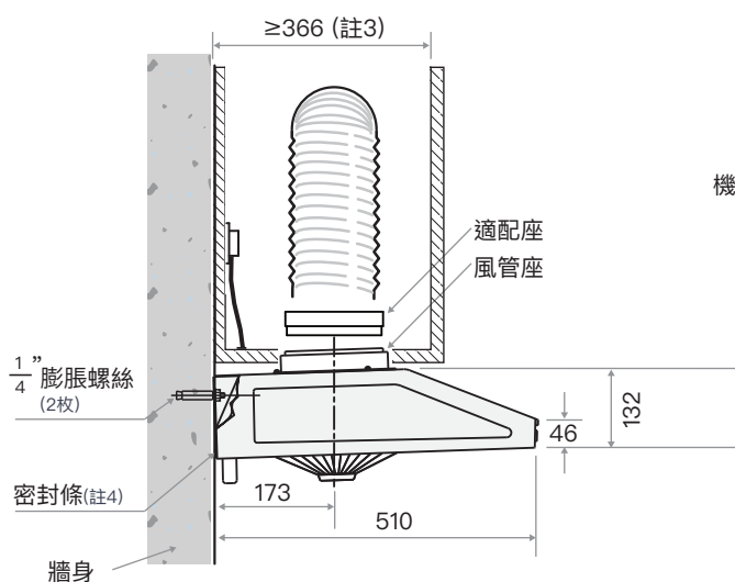
側視圖
