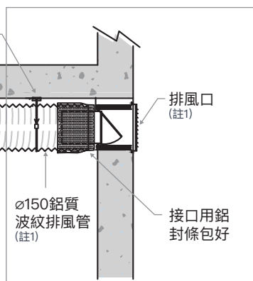
排風口在牆身
