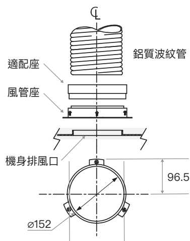
風管座
