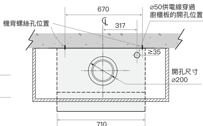
A-A 剖視圖
