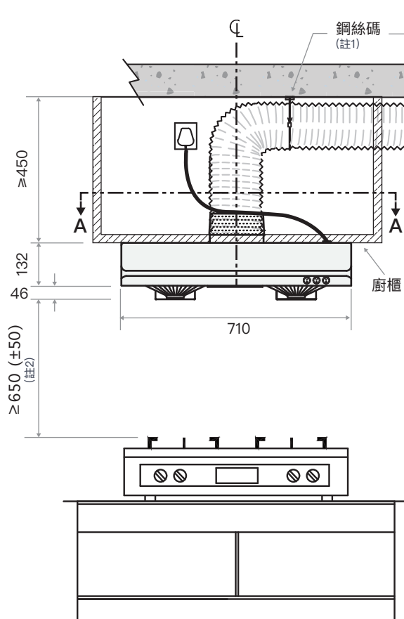
正視圖
