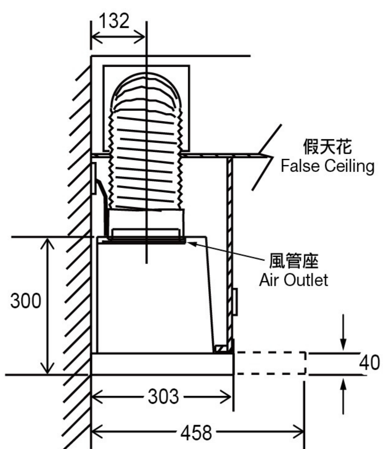
側視圖 Side View
