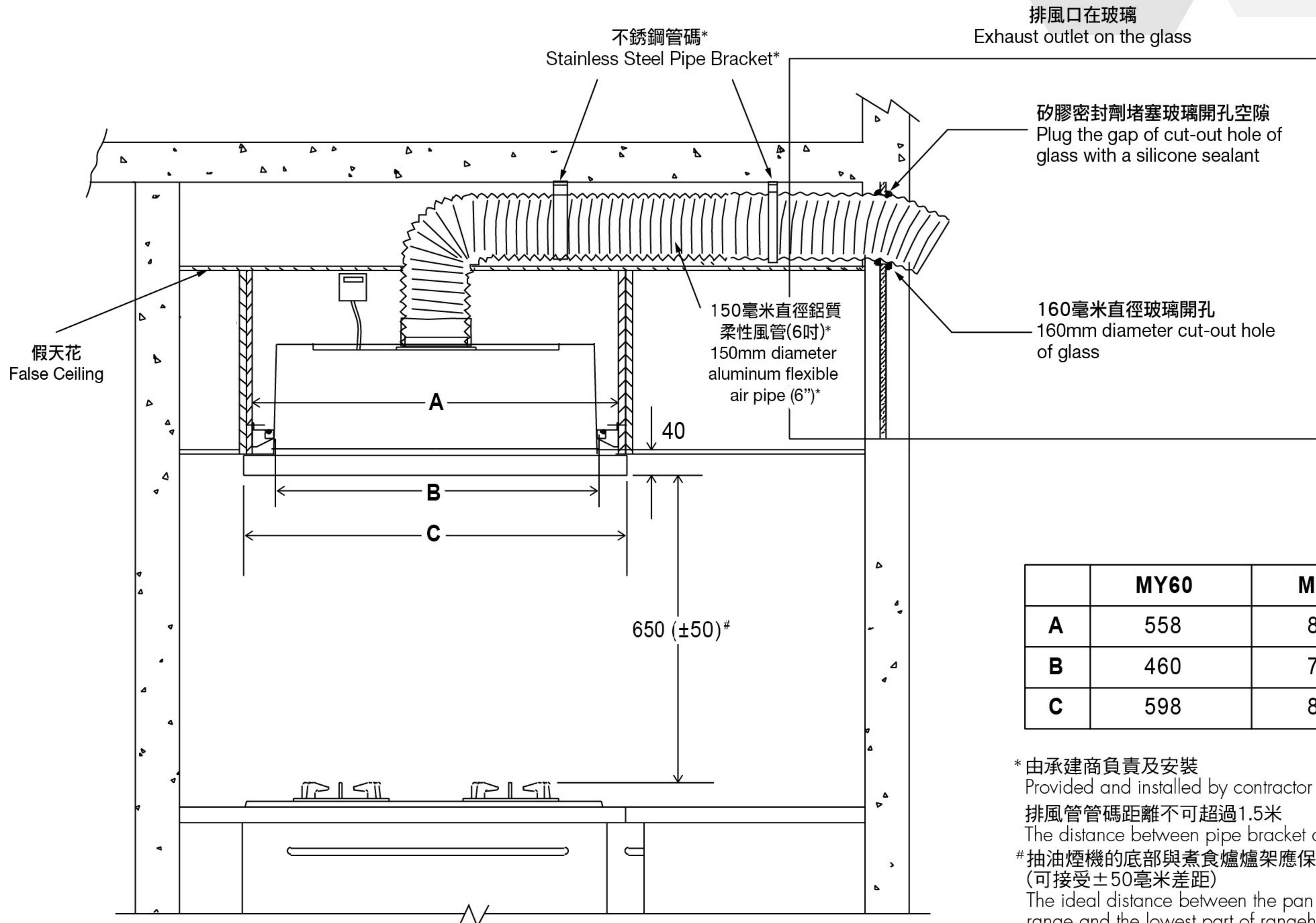
正視圖 Front View
